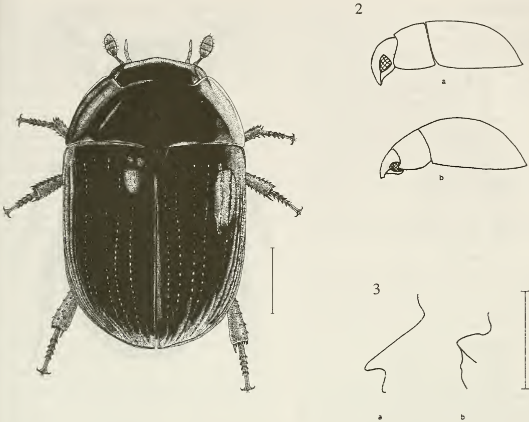
Figuras 1-3: 1. Andotypus perezdearcei n. sp., aspecto dorsal (escala = 1 mm). 2. Forma corporal, vista lateral, a: A. perezdearcei n. sp.; b: A. ashworthi Spangler. 3. Proceso mesosternal, vista lateral, a: A. ashworthi Spangler, b: A. perezdearcei n. sp. (escala = 0,5 mm)
