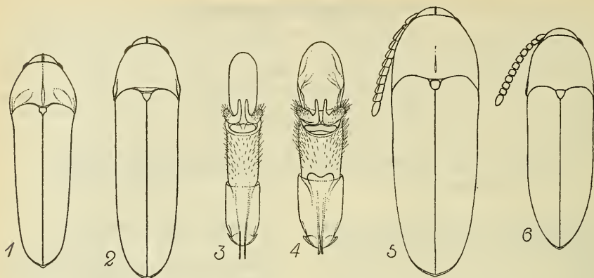
Fig. 1, silueta de Idiostarsus reedi carinatus nov. ssp.; fig. 2, silueta de Idiostarsus peñai nov. sp.; fig. 3, edeago de Idiostarsus reedi carinatus nov. ssp.; fig. 4, edeago de Idiostarsus peñai nov. sp.; fig. 5, silueta de Phanerochroeus australis nov. sp.; fig. 6, silueta de Xylophilus carinifrons nov. sp.
