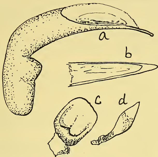
Pterostichus kuscheli Straneo. - Édéage. a) vue laterale; b) vue dorsale; c) d) styles.
