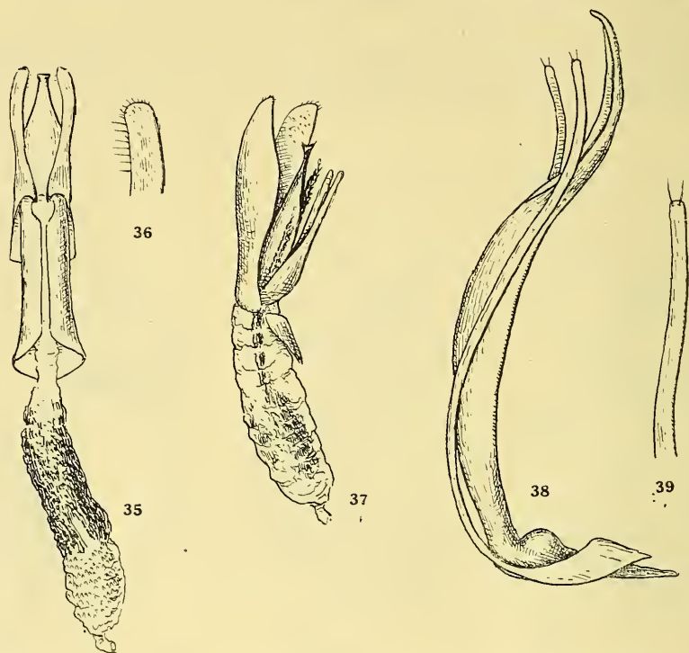
Fig. 35 à 39. Édages de Camiaridae de la Nouvelle-Zélande. — Fig. 35 et 36. Camiarus thoracicus Sharp. — Fig. 37. Camiarites convexus Sharp. — Fig. 38 et 39. Inocatops concinnus Broun.
