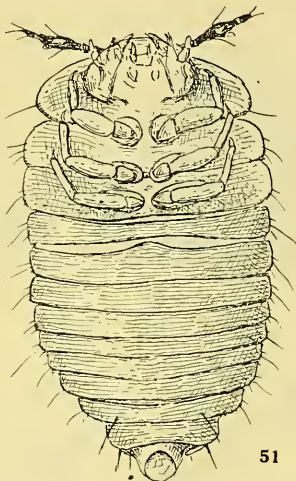
Fig. 50 et 51. Larve de Neocamiarus kuscheli n. sp. — Fig. 50. Face tergale. — Fig. 51. Face sternale.
