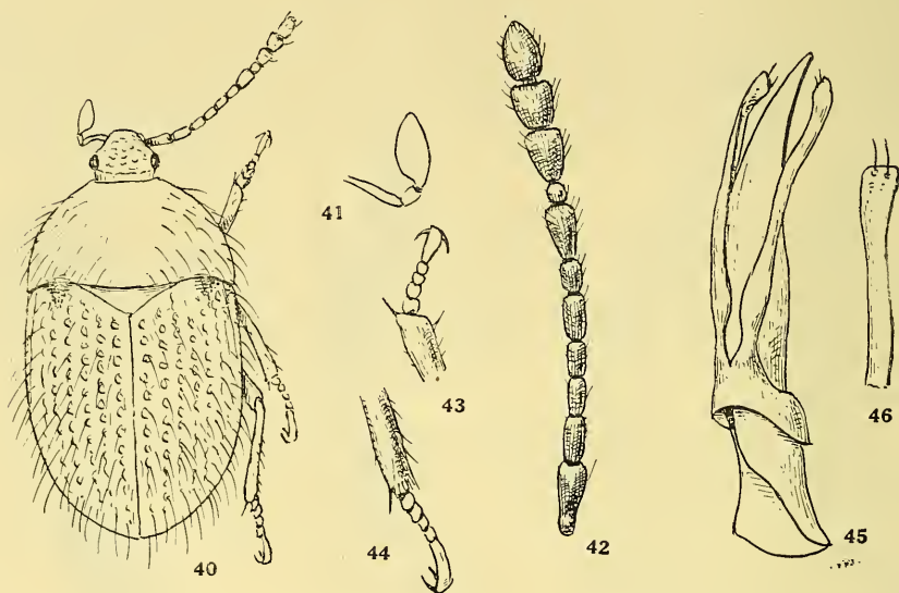
Fig. 40 à 46. Gen. Neocamarius nov. — Fig. 40. Silhouette du N. kuscheli n. sp., mâle, de Frutillar. — Fig. 41. Palpe maxillaire droit. — Fig. 42. Antenne droite. — Fig. 43. Tarse antérieur droit du mâle. — Fig. 44. Tarse postérieur droit. — Fig. 45. Édéage, face dorsale, \times 40 . — Fig. 46. Sommet du style gauche, face interne.
