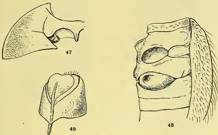
Fig. 47 à 49. Gen. Neocamiarus nov.; N. kuscheli n. sp. — Fig. 47. Pièces prosternales. — Fig. 48. Pièces méso- et métasternales. — Fig. 49. Segment génital, mâle, face sternale.
