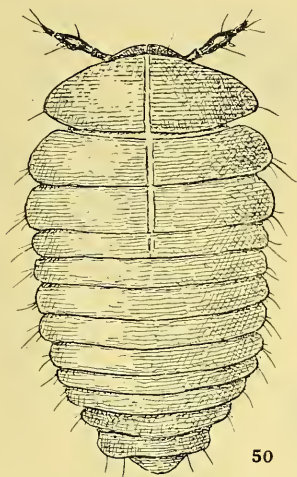
Fig. 50 et 51. Larve de Neocamiarus kuscheli n. sp. — Fig. 50. Face tergale. — Fig. 51. Face sternale.
