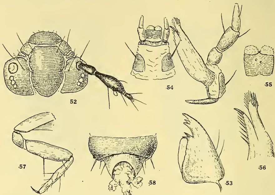
Fig. 52 à 58. Larve du Neocamiarus kuscheli n. sp. — Fig. 52. Tête, face tergale. — Fig. 53. Mandibule droite. — Fig. 54. Maxille gauche et pièces labiales. — Fig. 55. Langue plus grossie. — Fig. 56. Galéa et lacinia maxillaires plus grossies. — Fig. 57. Patte postérieure gauche, face sternale. — Fig. 58. Neuvième et dixième urites, face sternale.
